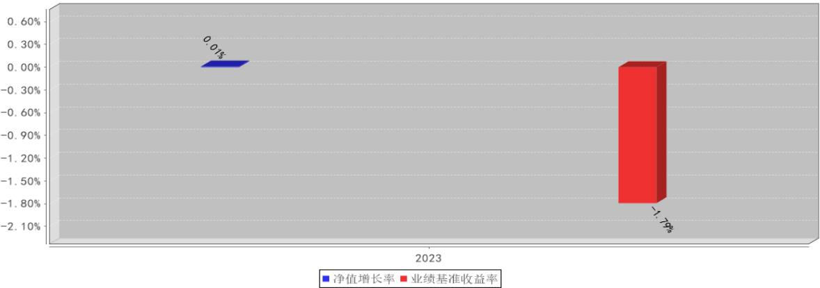
兴证全球兴晨六个月持有混合A基金每年净值增长率与同期业绩比较基准收益率的对比图（2023年12月31日）
