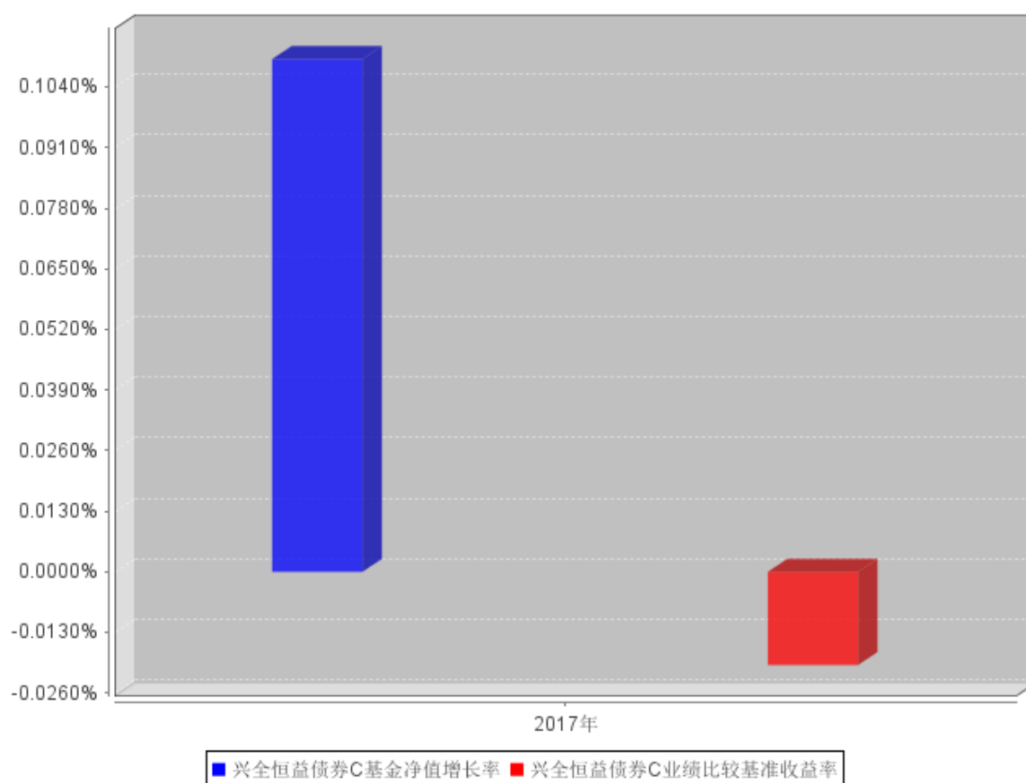
兴全恒益债券C自基金合同生效以来基金每年净值增长率及其与同期业绩比较基准收益率的对比图
